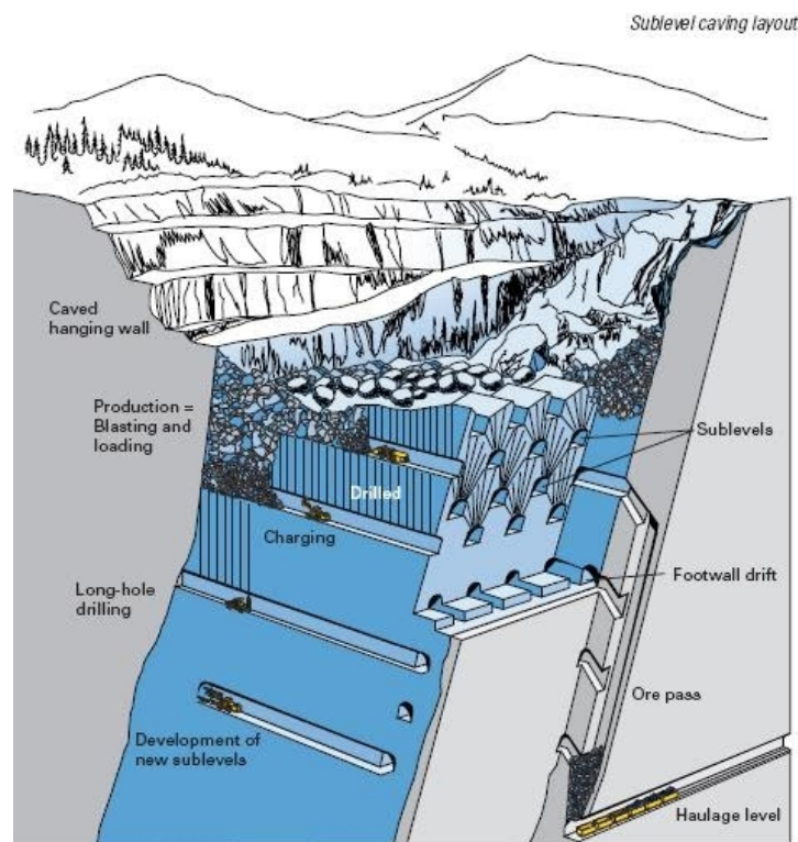
Sublevel longhole stoping
